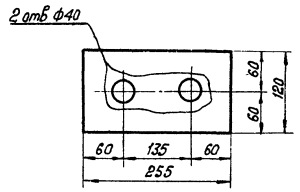
Деталь 3
