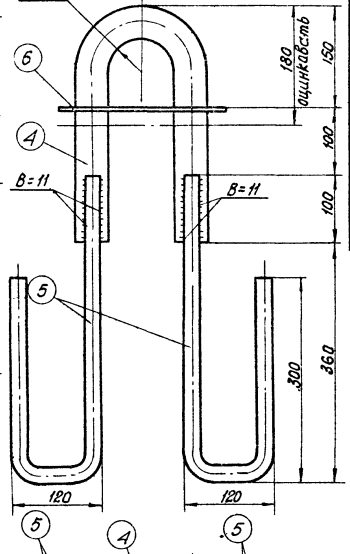
Деталь 6
