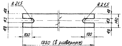
Деталь 7
