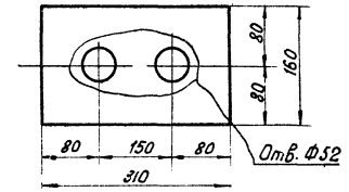
Деталь 6
