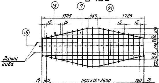
C-150
