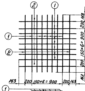
С-41
