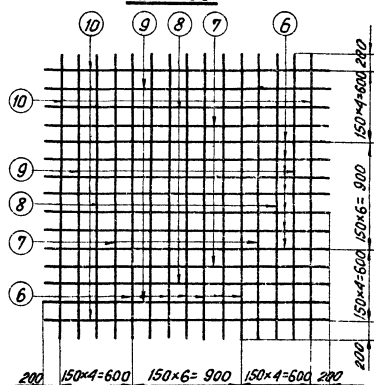
С-41
